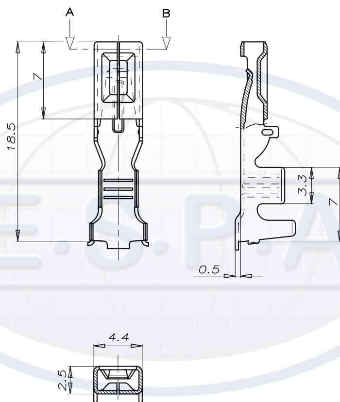
Section A-B
