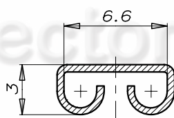
Section A-B
