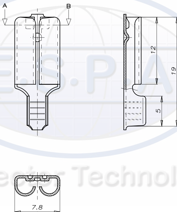
Section A-B
