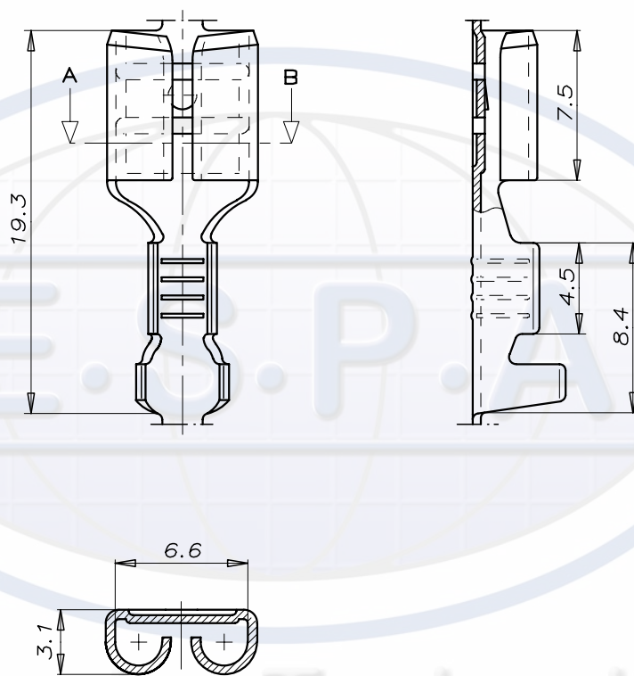
Section A-B
