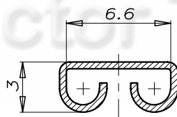
Section A-B
